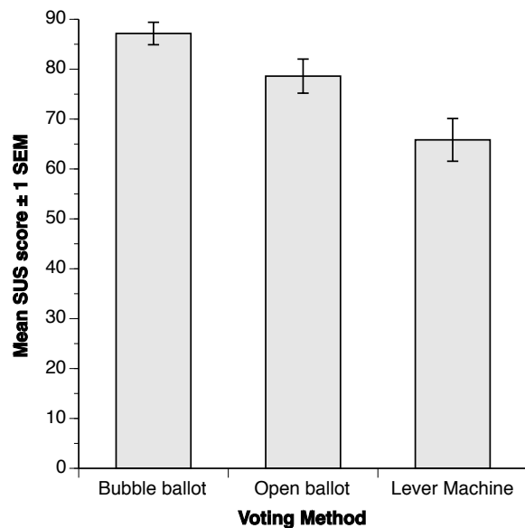
Figure 4. SUS scores
